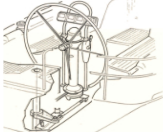
Beispiel für ein Cobra System
