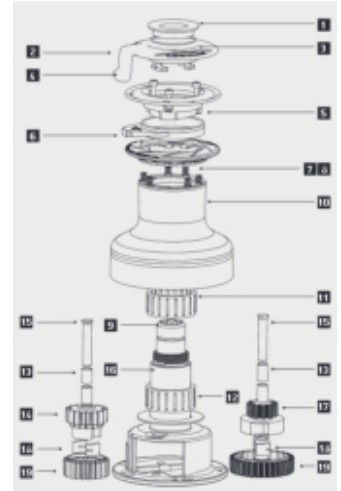
zerlegte EVO Winde
