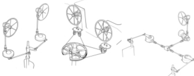
Beispielhafte Variationsmöglichkeiten für zwei Ruder und / oder zwei Steuerstände
