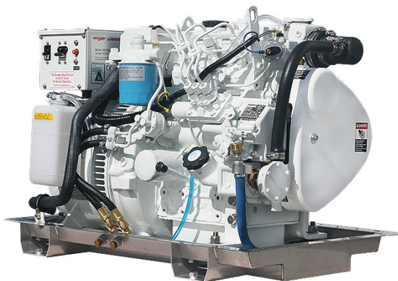
Modell M673L3 (5 kW/ 6 kW) - ohne Lärmschutzgehäuse
