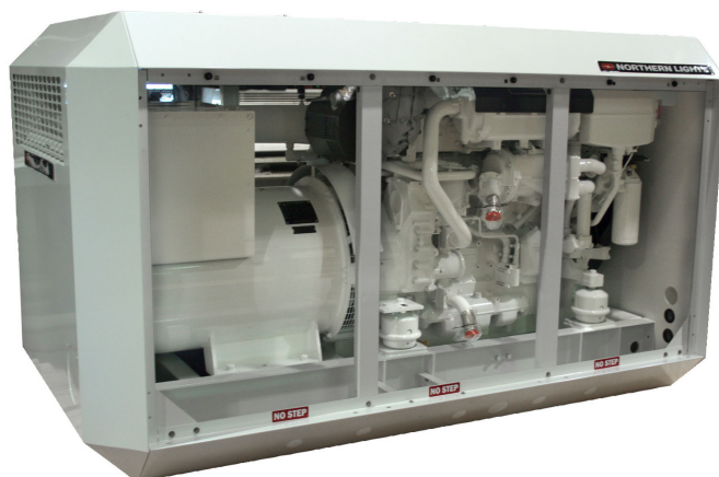
Modell M1305 – lieferbar von 185 kW bis 250 kW
